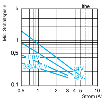
Kontakt mit Sprungfunktion
