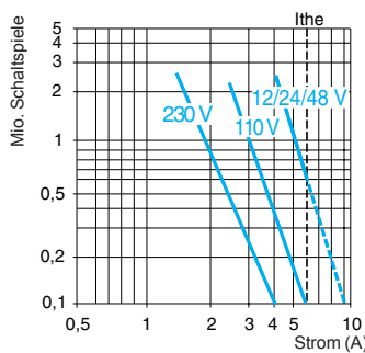
Kontakt ohne Sprungfunktion
